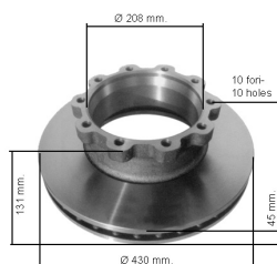
DISCO FRENO
