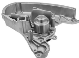
POMPA ACQUA
